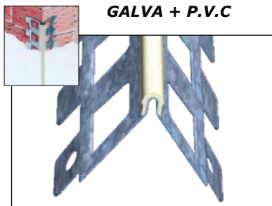
MONOCAPA GALVA + P.V.C
